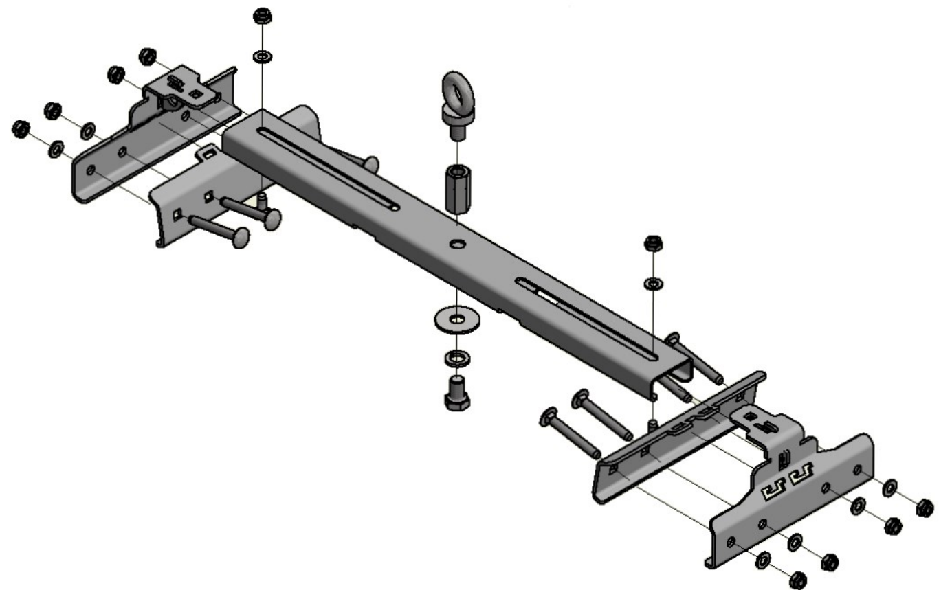
Variante mit Langmutter
