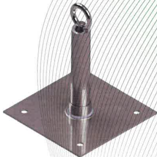
Bild 1: Anschlageinrichtung, Typ: Primo 3 AD ES BMP
