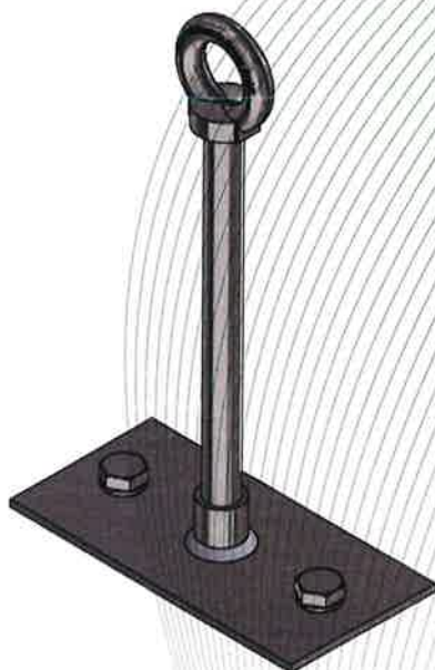
Bild 1: Anschlageinrichtung, Typ: Primo 2 ST BMP
